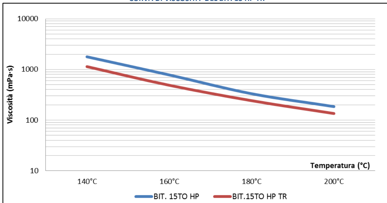
CURVA DI VISCOSITA' DEL BIT. 15 HP TR
